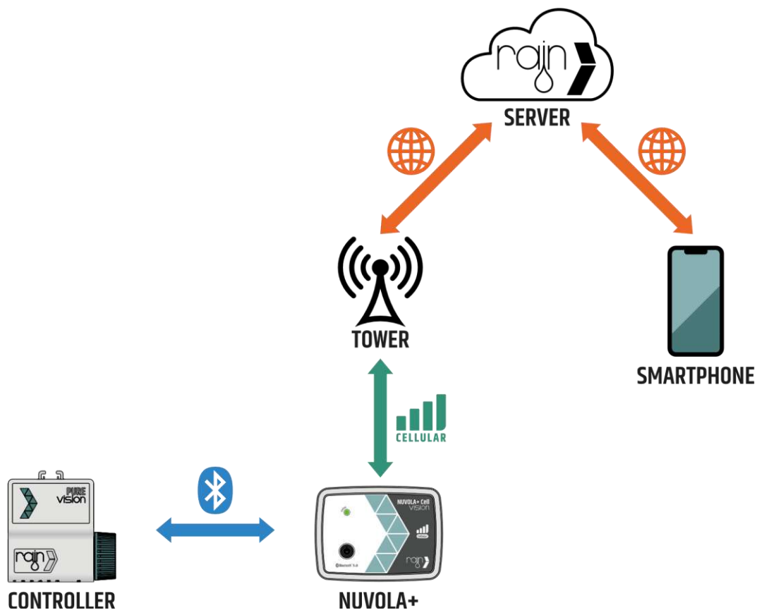
Struttura connessioni.
